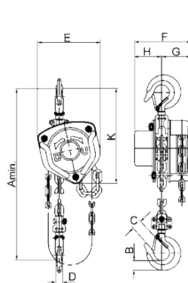
Silverline Stira S 500 - 2000 kg, single fall
