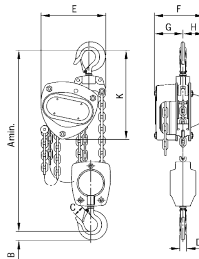
VSIII, 2000 - 5000 kg, double fall
