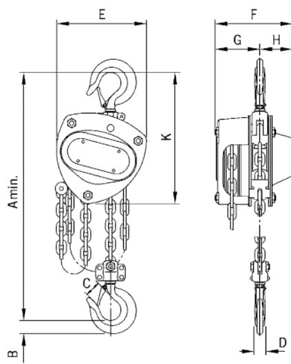
VSIII, 250 - 3000 kg, single fall
