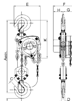
Silverline Stira S 3000 - 5000 kg, double fall
