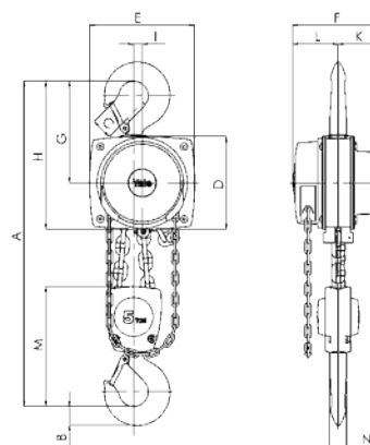
Yalelift 360, 5000 kg, double fall
