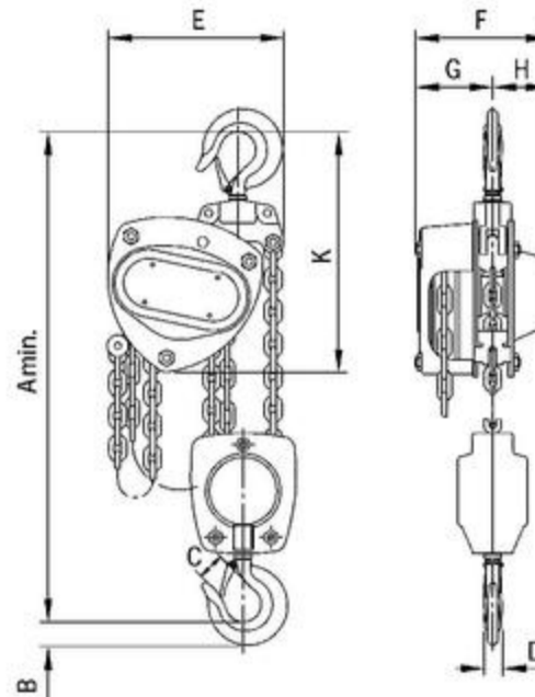
Model VSIII, 2000 - 5000 kg, double fall
